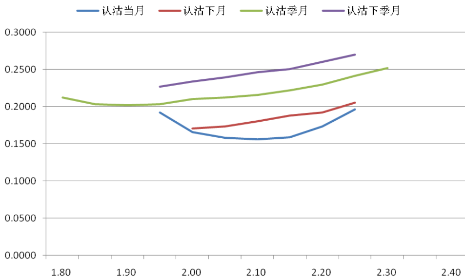
图 10：认沽期权隐含波动率微笑曲线（2016 年 7 月 1 日）
